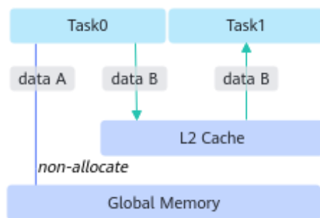
图4-10 Non-allocate (L2 hint) 典型应用场景示意图
