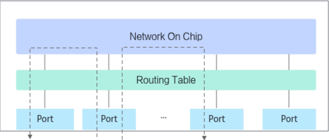
图4-15 UB On Chip Switch 转发示意图
