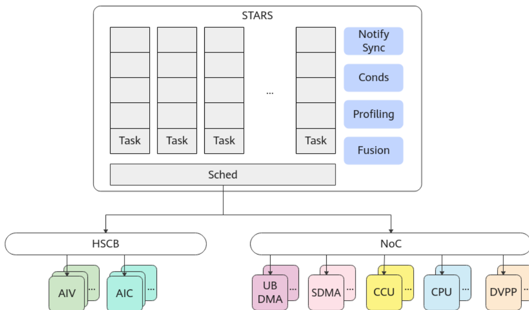
图4-11 STARS2.0 架构示意图
